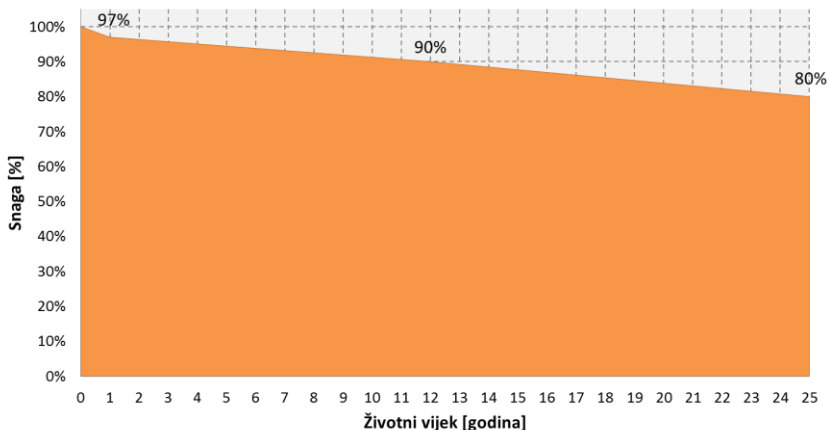
Slika 1. Graf linearne degradacije snage modula
